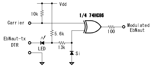
図 1: EX-OR による BPSK
